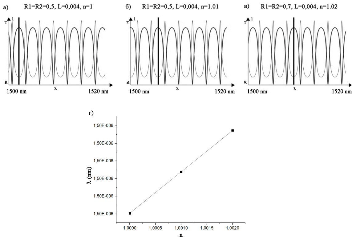
Рис. 4. График зависимости коэффициентов пропускания T и отражения R от длины волны \lambda , при R_1=R_2=0,5 , L=4*10^{-4} , для n=1 (а), n=1,01 (б), n=1,02 (в), график зависимости длины волны от показателя преломления (г)
