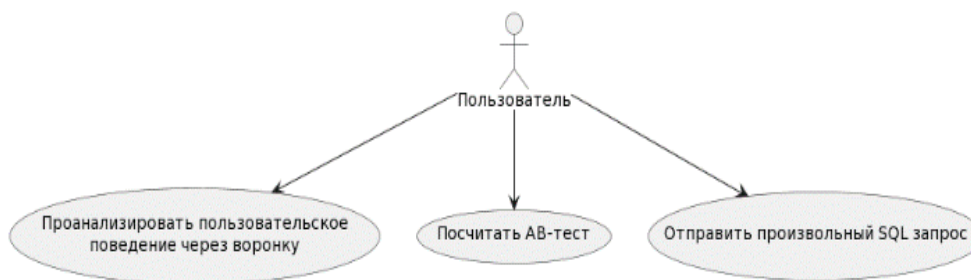
Рис. 1. Модель прецедентов
