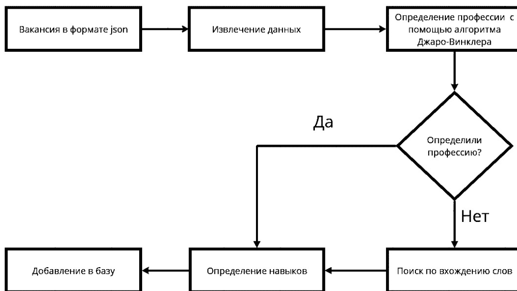
Рис. 1. Алгоритм обработки вакансий
