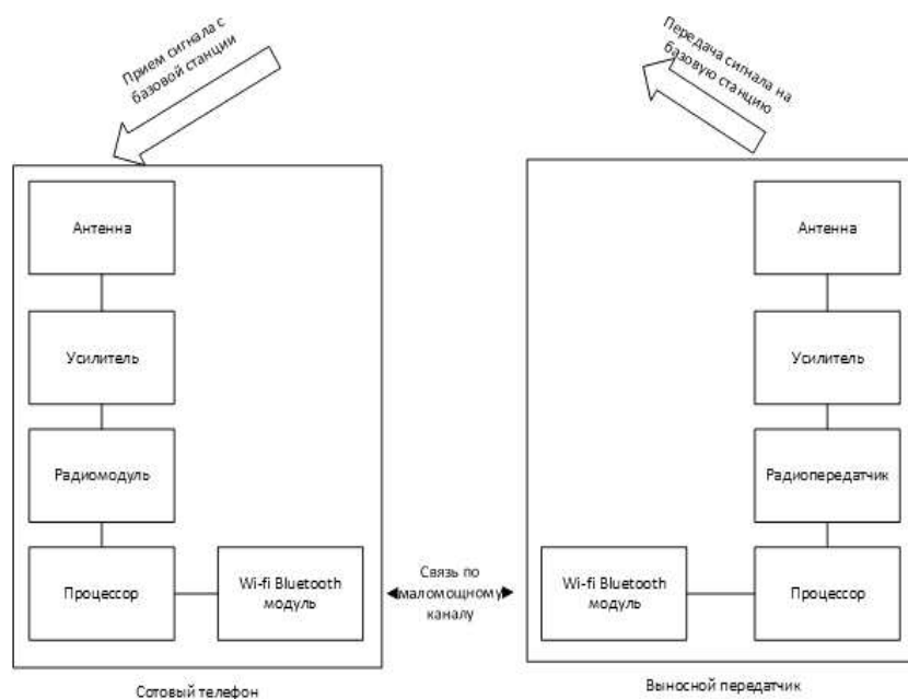
Рис. 2. Принцип работы сотового телефона с выносным передатчиком
