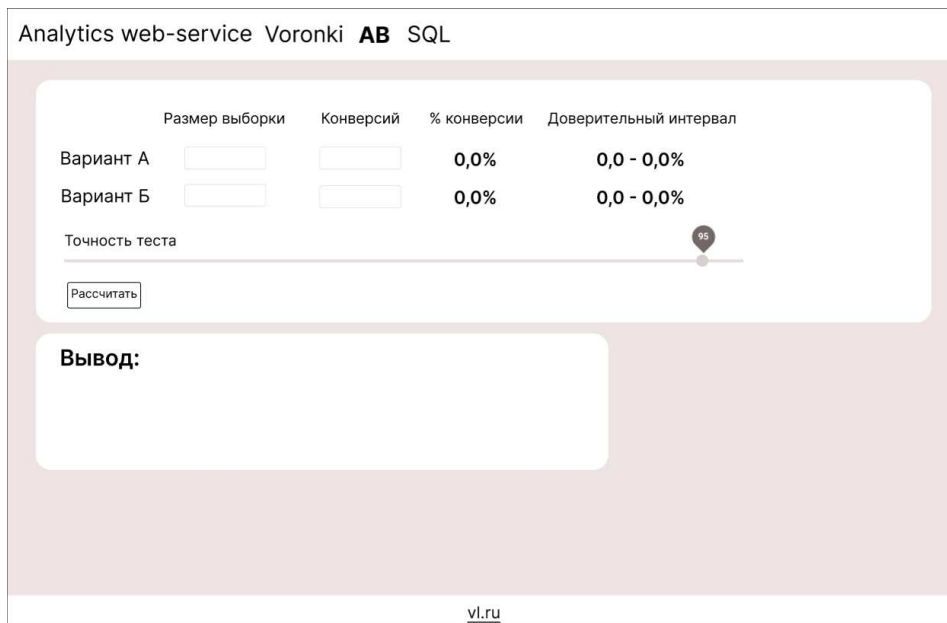
Рис. 3. Страница AB-теста
