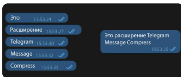
Рис. 1. Макет расширения
