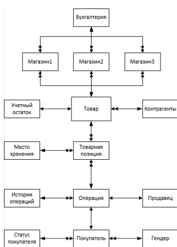
Рис. 4. Концептуальная модель БД
