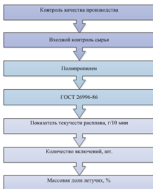
Рис. 3. Схема входного контроля материалов
