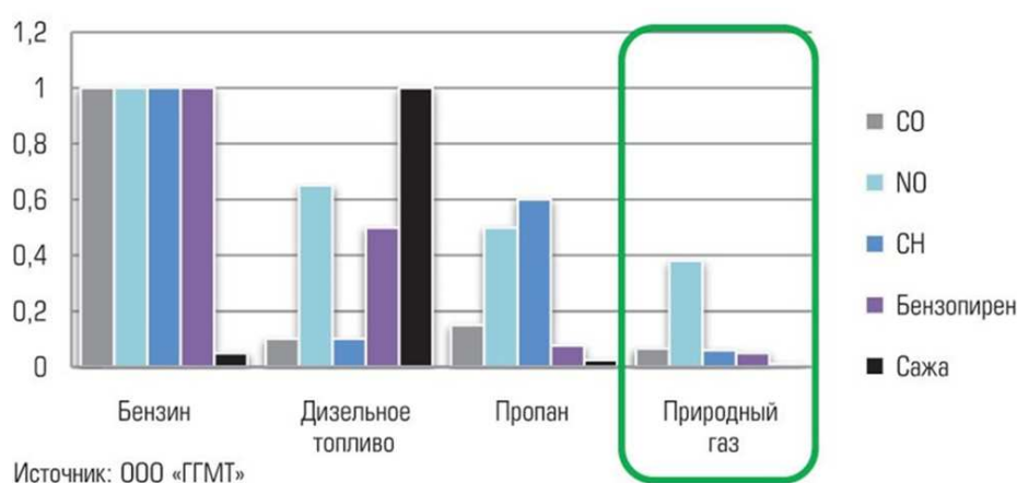
Рис. 1. Относительное содержание токсичных компонентов в отработанных газах
